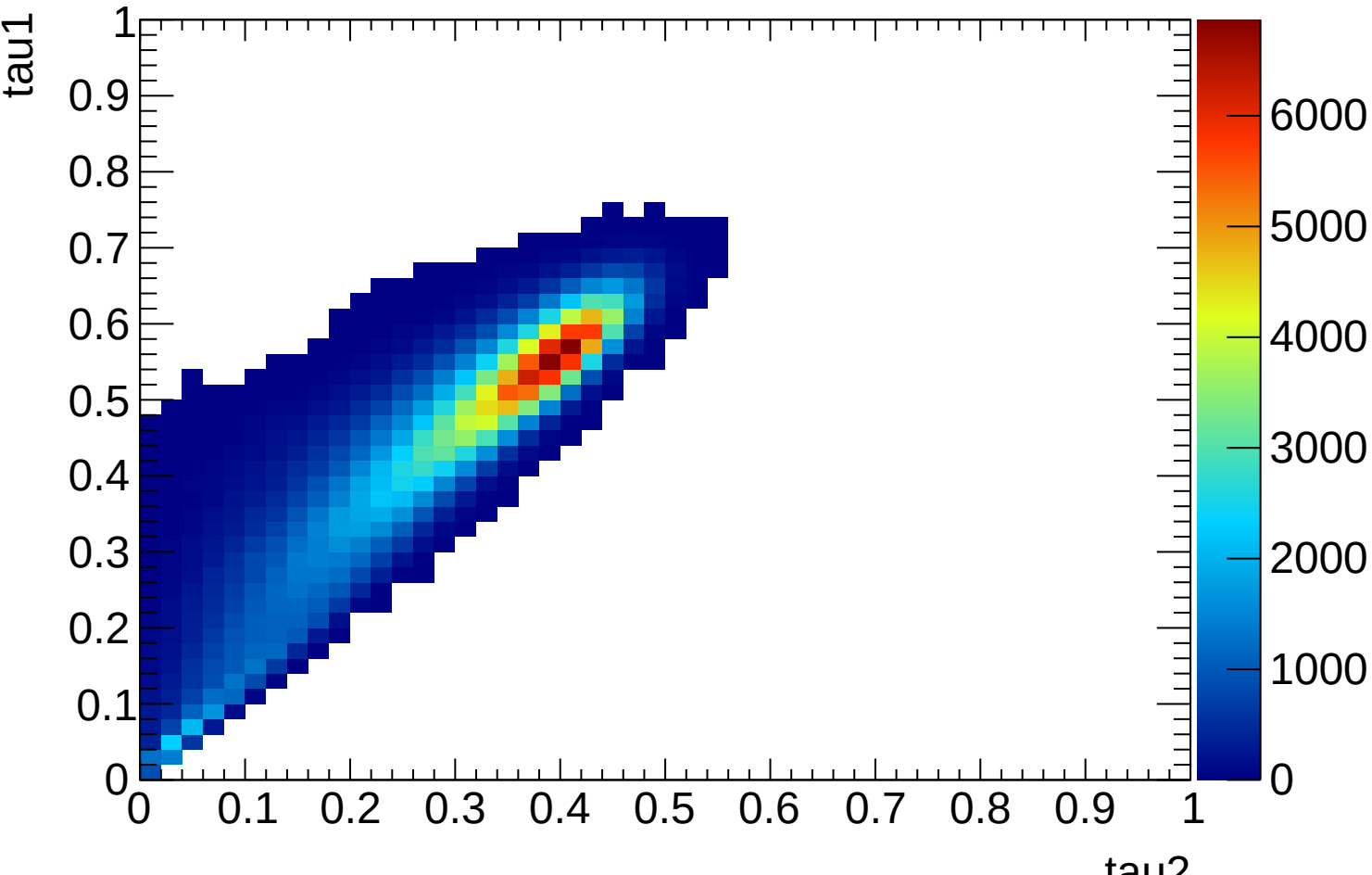
ak8jets_nJettinessTau1:ak8jets_nJettinessTau2
